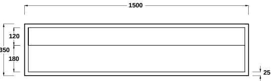
Prospetto frontale Front view
